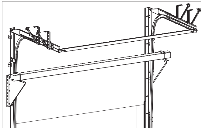
Рис. 19. Установка несущей балки
