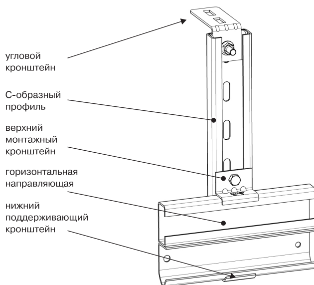
Рис. 18.1. Подвес
