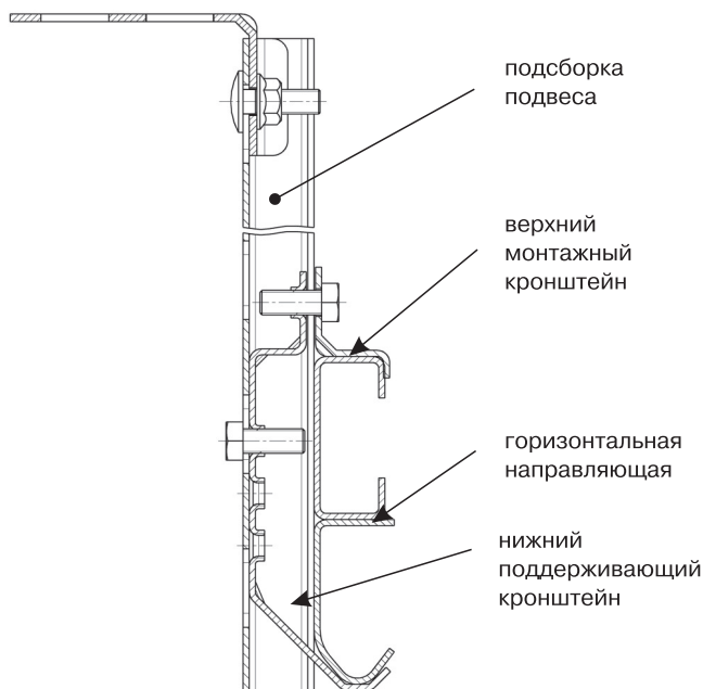
Рис. 18.3. Сборка подвеса
