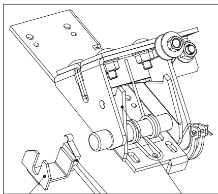
монтажный кронштейн микровыключатель выступ А
